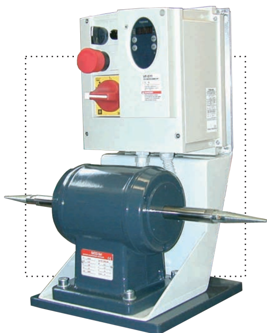
PLS 150K/2-Mv
